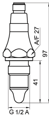
G 1/2 A DIN 3852-E (BCID: G51)
