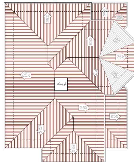
پلان بام
