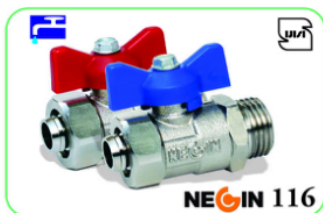
Model: NEGIN 116 مدل: نگین ۱۱۶ Size: 1/2 x 20 & 1/2 x 16 سایز: ۱/۲ x ۲۰ و ۱/۲ x ۱۶ PN: 25 Bar فشار کاری استاندارد: ۲۵ بار DN: 15 اندازه اسمی: ۱۵ Material: Brass جنس: برنج (روکش نیکل) Used: Non Gas مورد استفاده: غیر گازی
