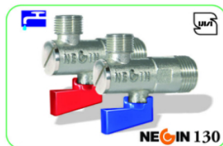
Model: NEGIN 130 مدل: نگین ۱۳۰ Size: 1/2 x 1/2 و 1/2 x 3/8 سایز: ۱/۲ x ۳/۸ و ۱/۲ x ۱/۲ PN: 25 Bar فشار کاری استاندارد: ۲۵ بار DN: 12 & 15 & 20 اندازه اسمی: ۱۲ و ۱۵ و ۲۰ Material: Brass جنس: برنج (روکش نیکل) Used: Non Gas مورد استفاده: غیر گازی
