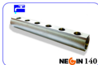
Model: NEGIN 140 مدل: نگین ۱۴۰ Size: G 3/4".....1-1/4" سایز: ۳/۴ اینچ.....۱.۱/۴ اینچ PN: 25 Bar فشار کاری استاندارد: ۲۵ بار DN: 20.....32 اندازه اسمی: ۲۰.....۳۲ Material: Brass جنس: برنج (روکش برنج) Used: Non Gas مورد استفاده: غیر گازی
