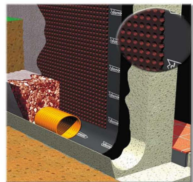
هدایت آب زهکشی شده به سوی لوله های زهکش
