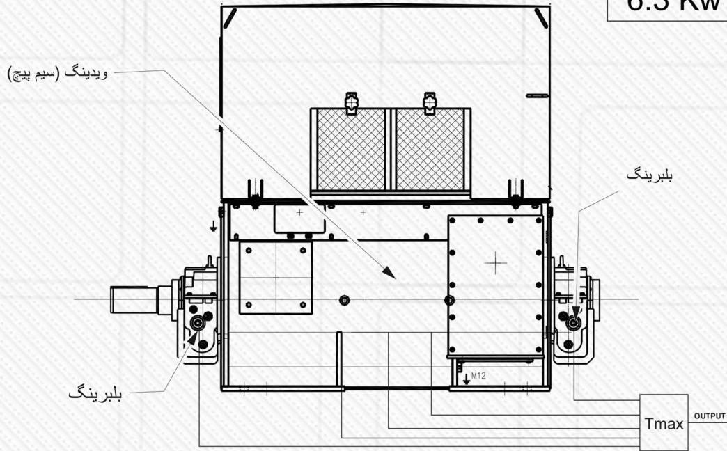
اندازه گیری سه عدد ویدینگ (سیم پیچ) و دو عدد بلبرینگ
