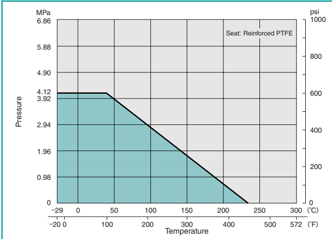
Type 600 : SCKT/UTKM
