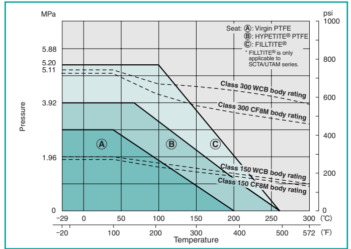
150 UTBM : 5" & 6"* 150/300 SCTA/UTAM : 8" & 10"
