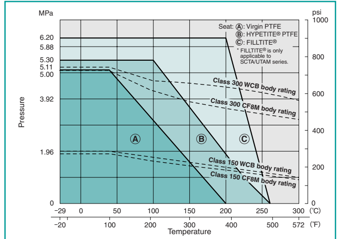
150 UTBM : 5" & 6"* 150/300 SCTA/UTAM : 8" & 10"
