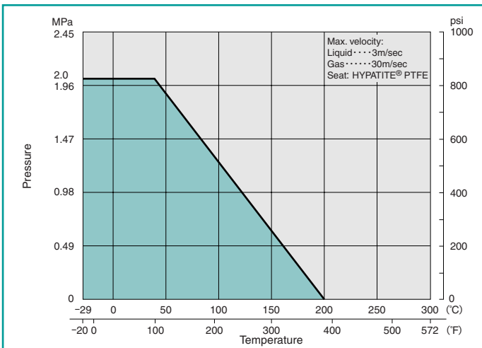
Type 800 : UTH4LM/4TM
