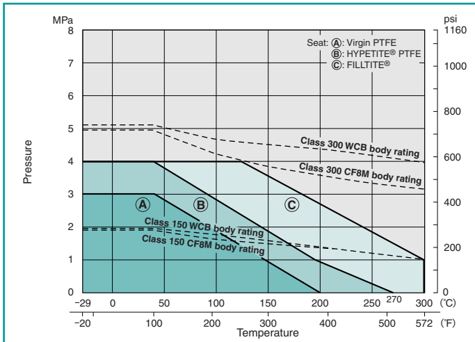
150/300 UTDZM/SCTDZ: 8", 10"
