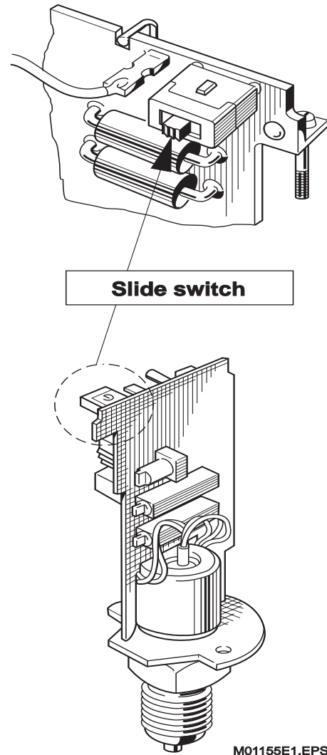
Bild 19. Position of the slide switch e.g. AMD 200
